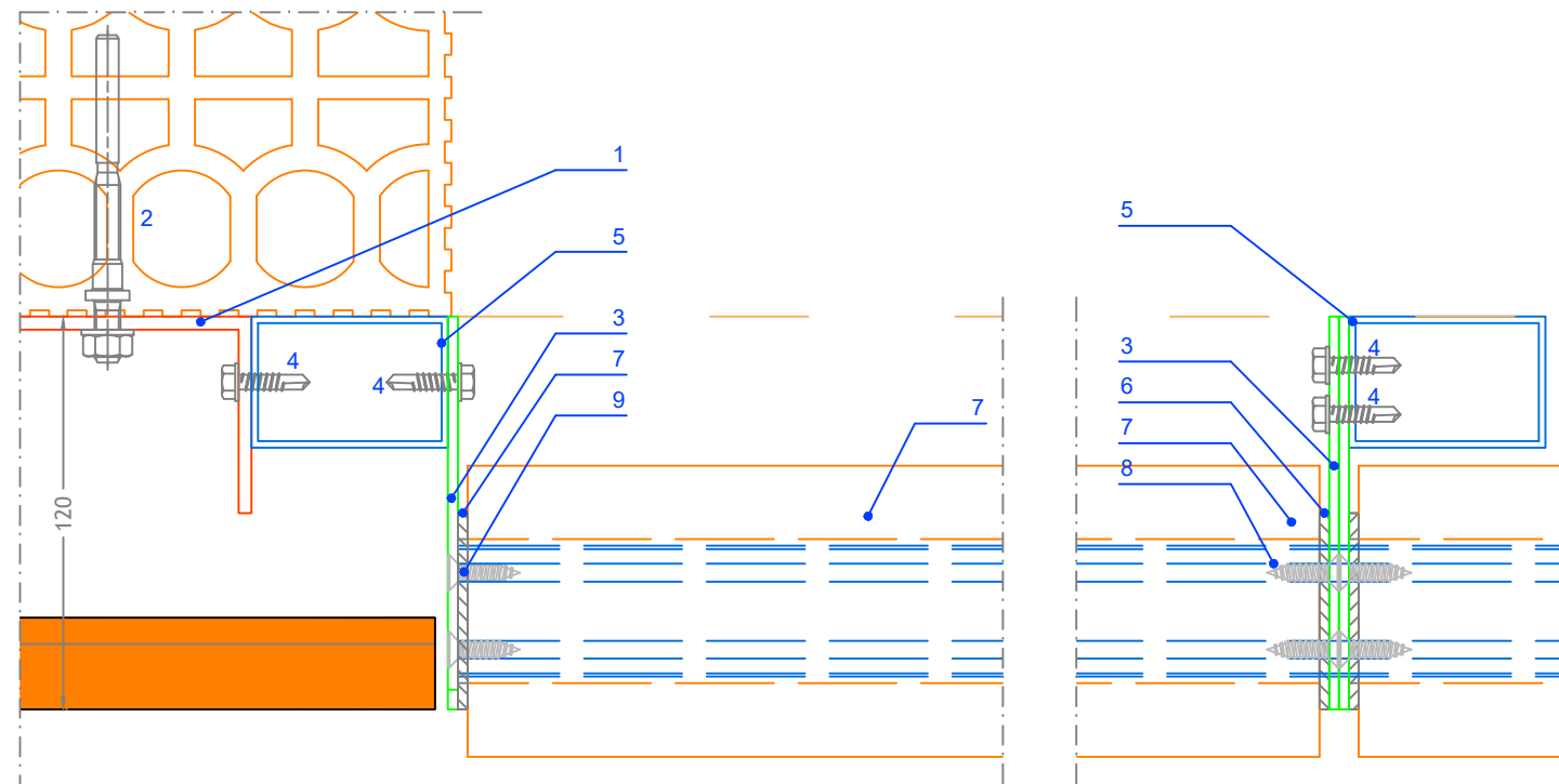
DETAIL 1 SCALE: 1/2.5
