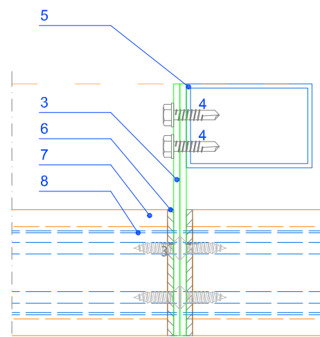
DETAIL 2 scale: 1/2.5
