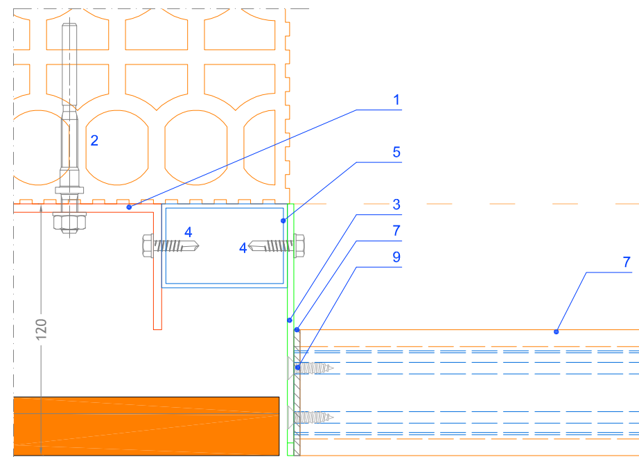
DETAIL 1 scale: 1/2.5
