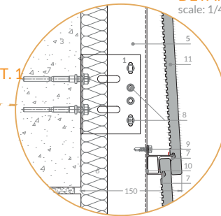
DETAIL 1 scale: 1/4
