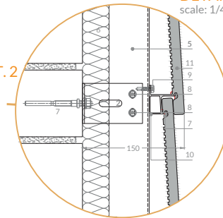
DETAIL 2 scale: 1/4
